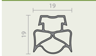
RP362 solid EPDM
