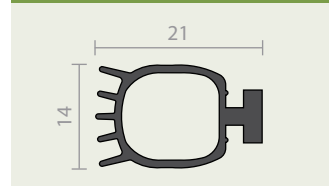
RP362 solid EPDM
